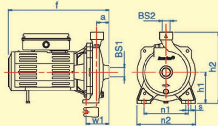
WCH-755S / WCH-1105S
