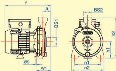
ACH-375S
